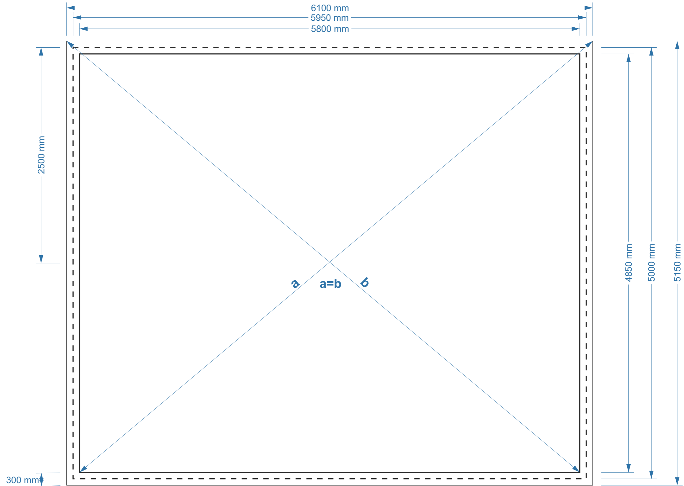
Fundație tip centură beton
