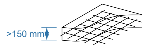
Fundație tip placă beton (plasă sudată Ø6mm, ochi 100X100mm)
