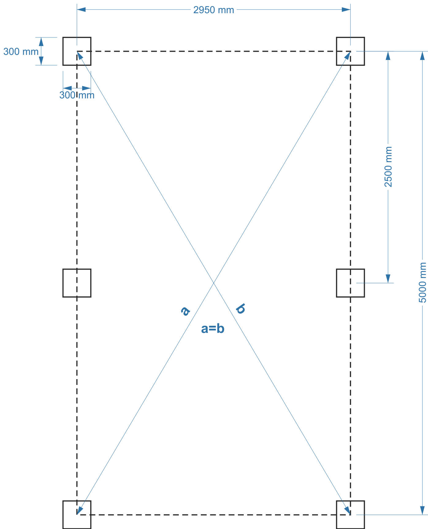
Amplasarea garajului metalic pe fundația tip stâlpi de beton
