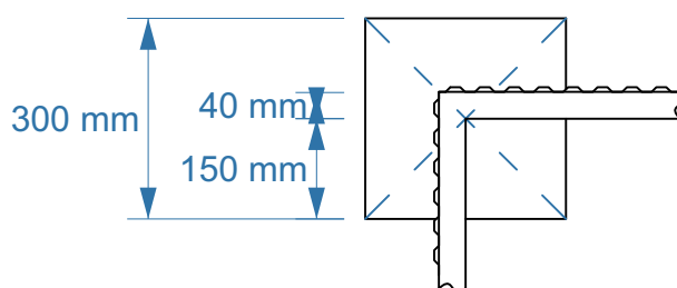
Amplasarea garajului metalic pe fundația tip stâlpi de beton
